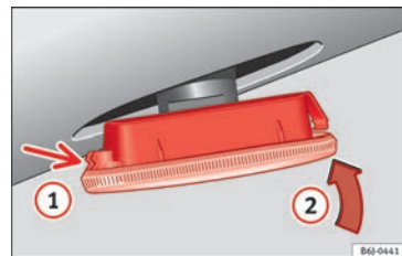
Fig. 193 Intermitente lateral.
