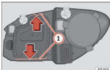
Fig. 178 Luz de cruce.
