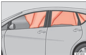
Fig. 18 Airbags para la cabeza inflados.
