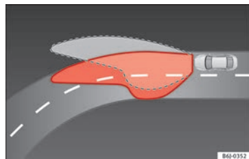
Fig. 62 Iluminación de la curva con faros autodireccionables.
