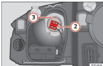
Fig. 179 Luz de cruce.
