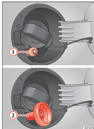
Fig. 140 Tapa del depósito abierta con boca de carga de GLP y adaptador.
