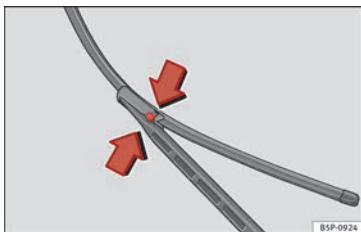
Fig. 170 Cambio de las escobillas del limpiaparabrisas.
