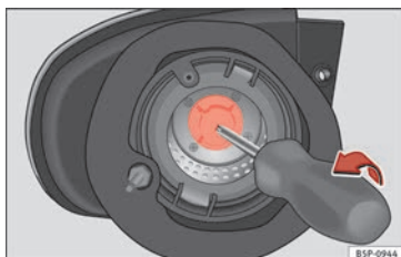
Fig. 187 Luz intermitente.
