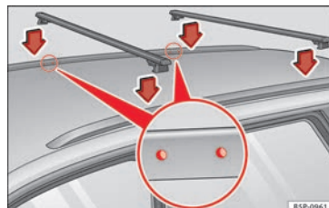
Fig. 113 Modelo Altea XL/Altea Freetrack: puntos de fijación para el portaequipajes del techo.
