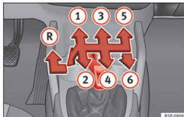
Fig. 124 Detalle de la consola central: esquema de un cambio manual de 5 o 6 marchas.
