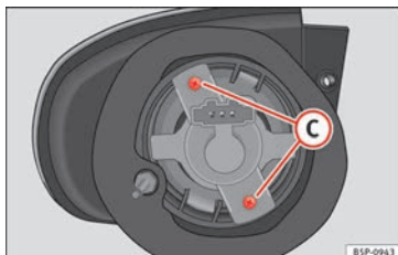
Fig. 186 Luz intermitente.
