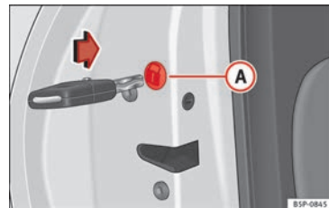
Fig. 167 Cierre de emergencia de las puertas.
