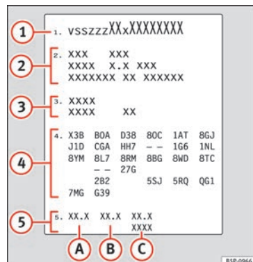
Fig. 202 Portadatos del vehículo (maletero).
