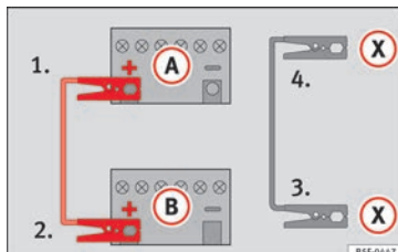
Fig. 164 Esquema de conexión para vehículos con sistema Start-Stop.
