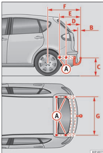
Fig. 138 Puntos de fijación del dispositivo de remolque.
