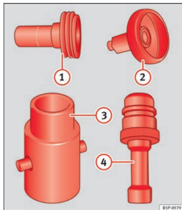
Fig. 142 Cuadro general de los adaptadores para la boca de carga de GLP.
